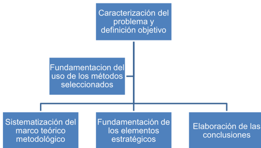
Figura 2: Esquema metodológico
